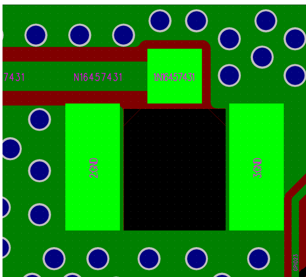
图 19: ESP32 系列芯片 IPEX 版图设计
