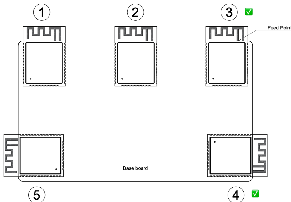
图 23: ESP32 系列模组 (天线馈点在右侧) 在底板上的位置示意图
