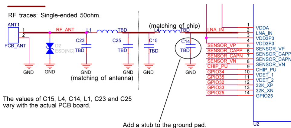
图 7: ESP32 系列芯片射频匹配电路图
